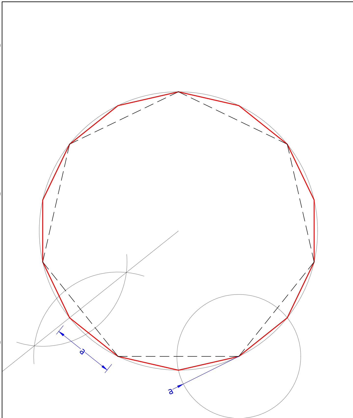
Näherungskonstruktion aus Siebeneck
